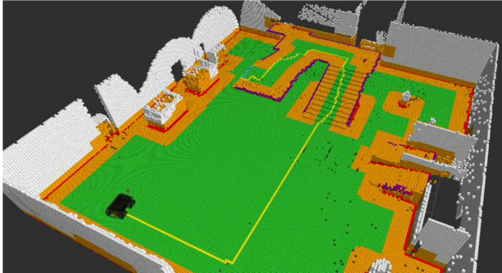
Abb. 8.3.2: Befahrbarkeitsanalyse und Pfadplanung für 3D Exploration.
