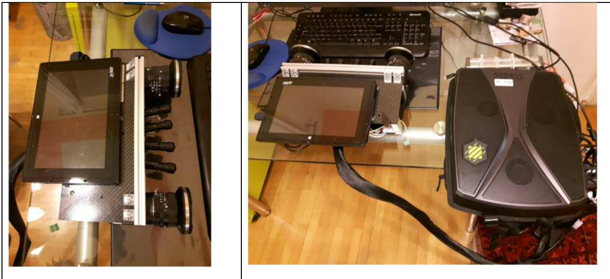
Abb. 6.1.3: Mobiles Stereosystem zur Datenaufnahme.
